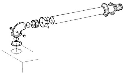
SCARICO COASSIALE ORIZZONTALE Ø 100 mm
