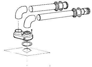
SCARICO SDOPPIATO Ø 80 mm con scarico condensa
