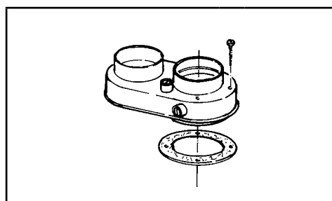
SDOPPIATORE con scarico condensa
