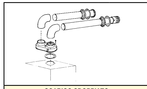
SCARICO SDOPPIATO Ø 80 mm con scarico condensa
