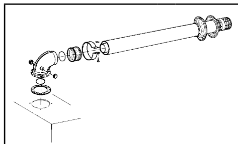
SCARICO COASSIALE ORIZZONTALE Ø 100 mm (mt 1)
